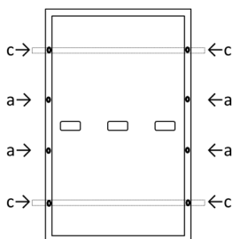
Rys. B1: Położenie otworów montażowych
